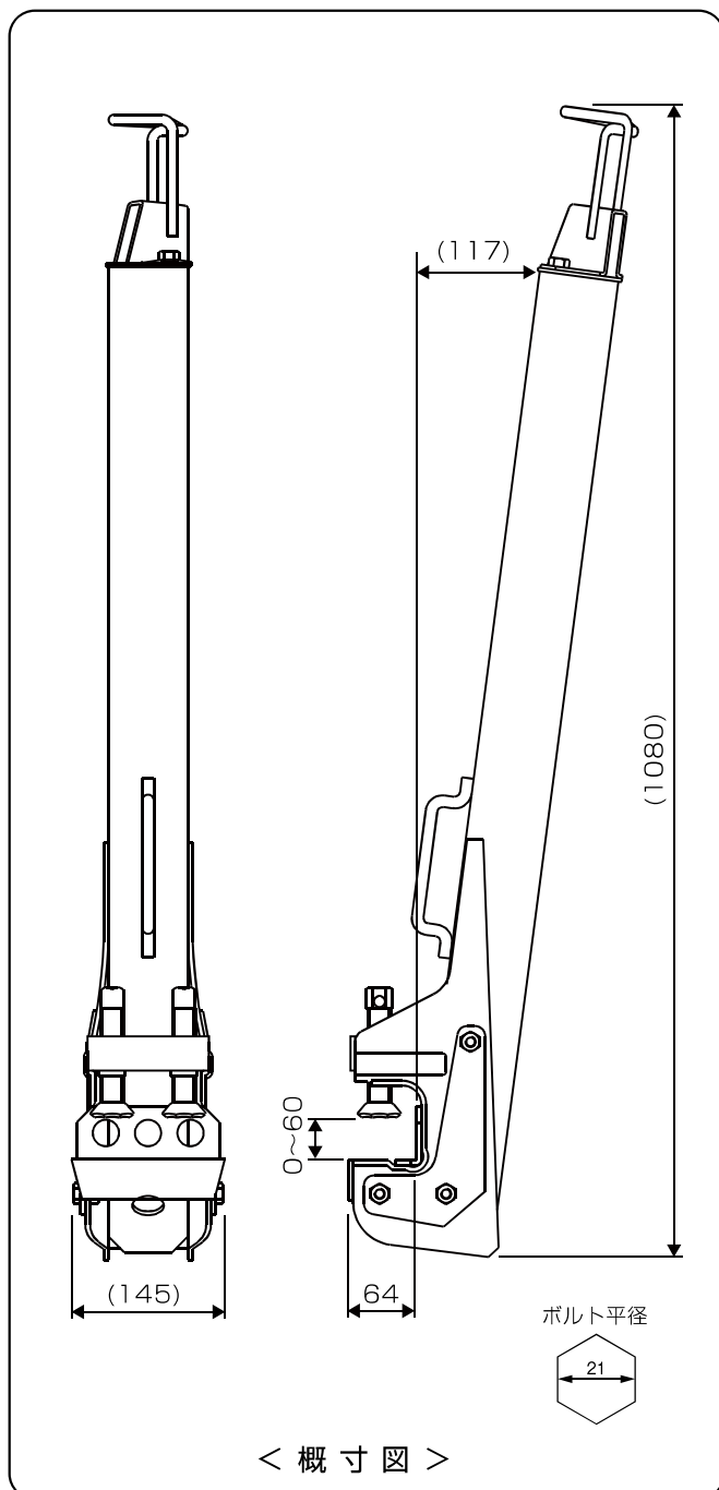
KS 親網支柱兼用C型
