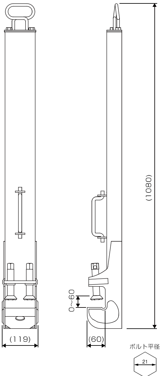
< 概 寸 図 >
